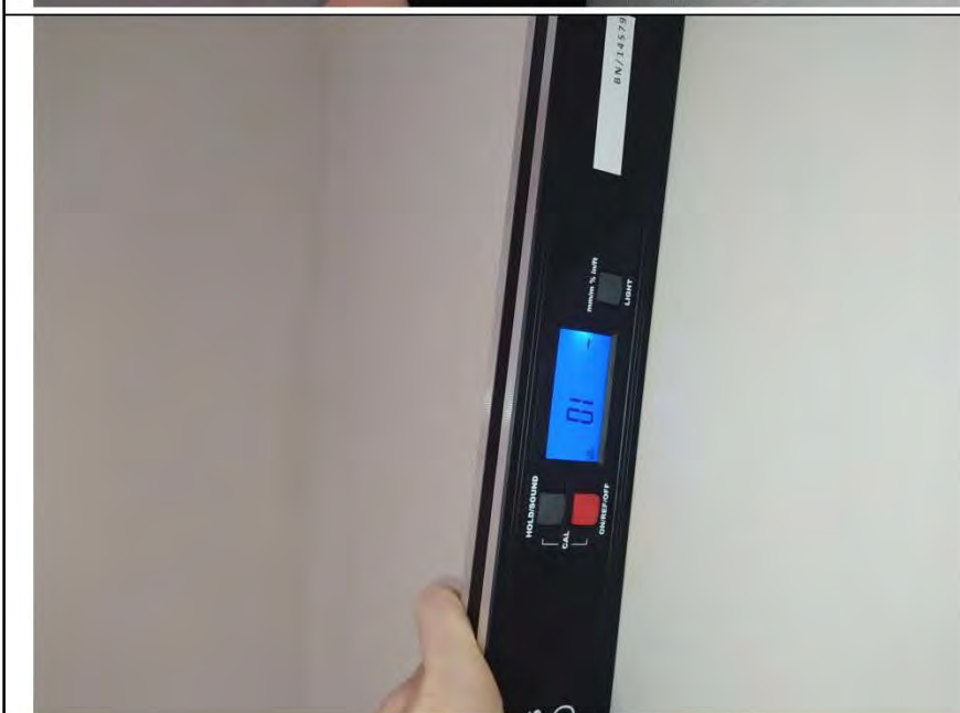
Фото №9. Измерение уровня стен в ванной комнате.
