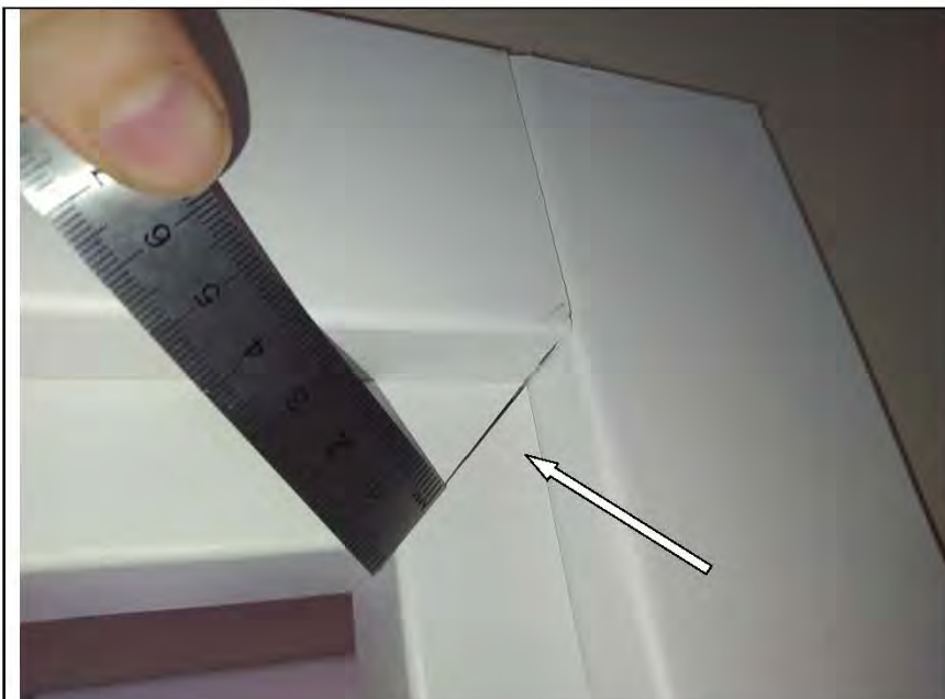
Фото №34. Элементы дверного блока соединены не надежно в ванной комнате.
