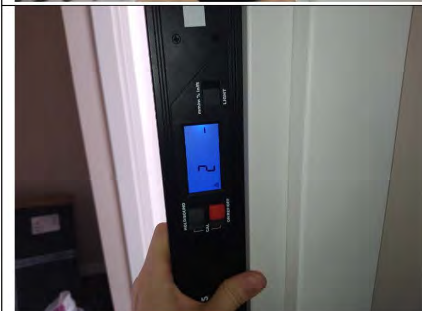
Фото №29. Отклонение коробки дверного блока в ванной комнате.
